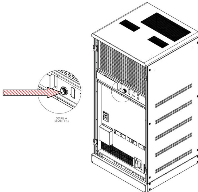
Маршрут прокладки кабеля связи для ИБП Keor T 120 кВА
