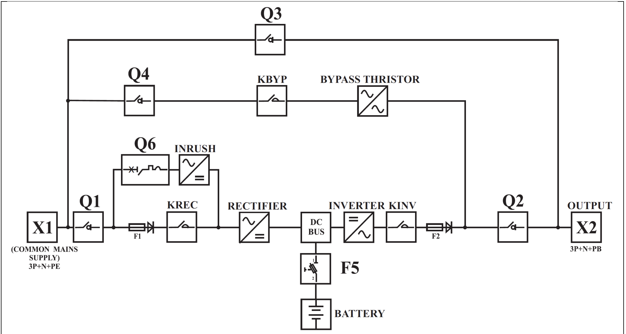
СХЕМА ОДИНОЧНОГО ИБП С ОБЩИМ ВВОДОМ ВЫПРЯМИТЕЛЯ И БАЙПАСА (80-120 кВА)
